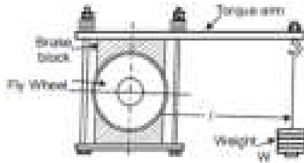
Fig. 29. Prony brake
