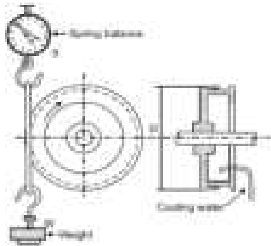
Fig. 30. Rope brake
